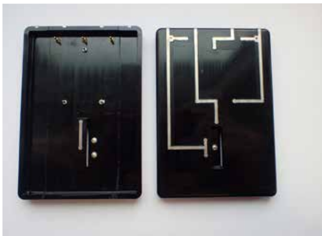
Abbildung 1: Mit dem Metalldirekteinspritzen gefertigter Demonstrator
