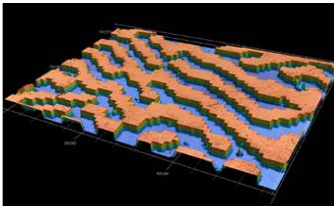
Abbildung 1: Diffraktives optisches Element (DoE, Struktur in Silikon)
