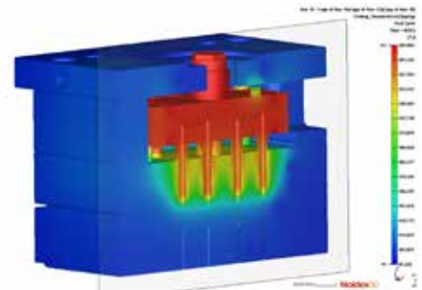
Abbildung 1: Prozesssimulation des Werkzeuges
