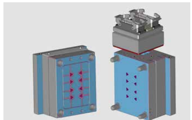
Abbildung 2: Werkzeugkonstruktion
