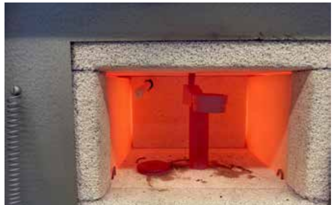
Abbildung 1: Prüfstand zur Analyse der Chrommigration im Ofen bei 800 °C
