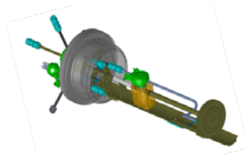
Abbildung 2: Verdampfer für die sequenzielle Verdampfung von zugeführtem Präkursor
