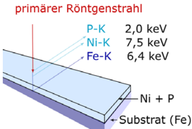
Abbildung 1: direkte Bestimmung des P-Anteils in NiP-Schichten
