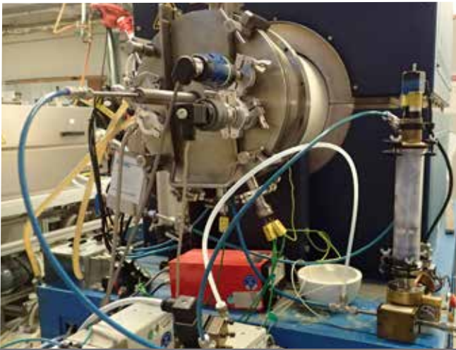
Abbildung 2: CVD 1 mit installiertem System zur Prozessierung von Feststoffprecursoren
