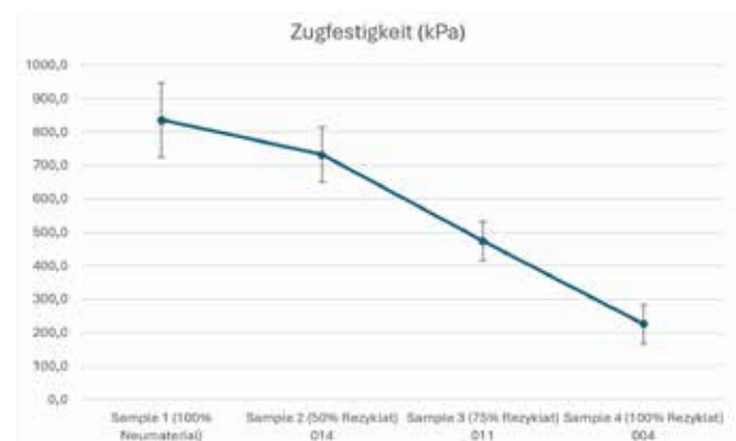
Abbildung 2: Zugfestigkeit nach ISO 1798 der Recyclingstufe 1 (ARPRO 5135) aus Plattenmaterial
