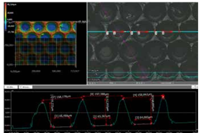
Abbildung 2: hexagonale Struktur, Abformung in Glas, Ermittlung von charakteristischen Oberflächenmaßen.
