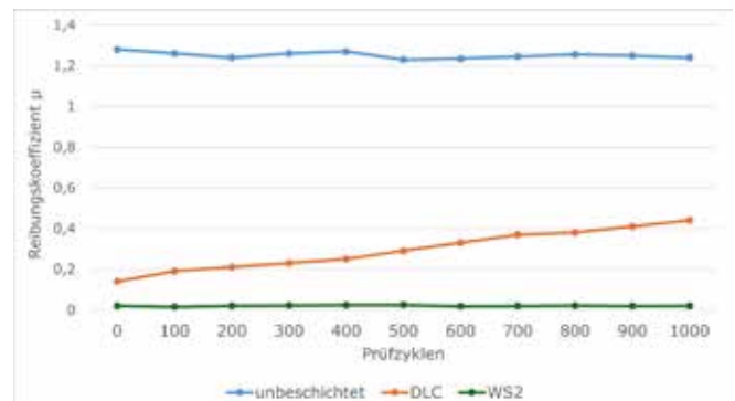
Abbildung 2: Bei 135°C ermittelte Reibungskoeffizienten auf Auswerfern aus 1.2210 im Vergleich: mit Wolframsulfid, DLC und unbeschichtet.
