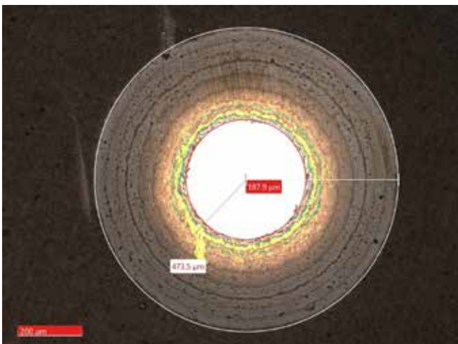
Abbildung 1: Analyse der Schichtdicke
