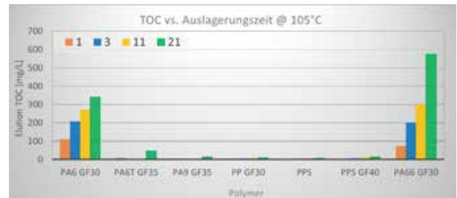
Abbildung 1: TOC-Werte in Abhängigkeit der Auslagerungszeit (in Tagen) und des Materials bei 105°C
