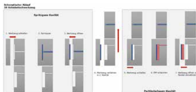
Abbildung 1: Schematische Darstellung des One-Shot Verfahrens mittels Schiebetischwerkzeug
