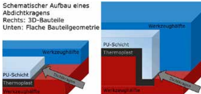
Abbildung 1: Kunststoffbauteil mit Quetschkante beim IMC
