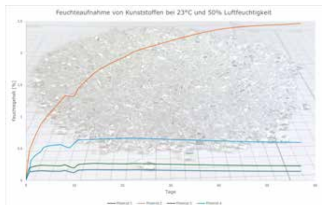
Abbildung 2: Feuchtaufnahme verschiedener Granulate
