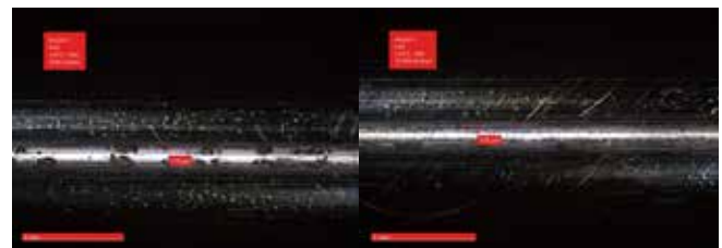
Abbildung 1: Reibspur eines mit WS 2 beschichteten HSS-Auswerferstiftes nach Reibprüfung bei 135 °C: nach 5000 Zyklen links und nach 10.000 Zyklen rechts
